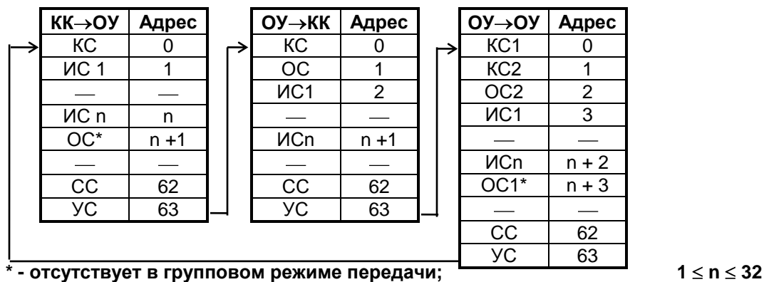
Рис. 4. Пример структуры блока памяти в режиме МК.
