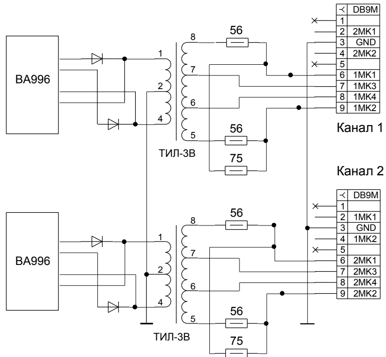
Рис. 15. Подключение устройства к линии передачи информации.
