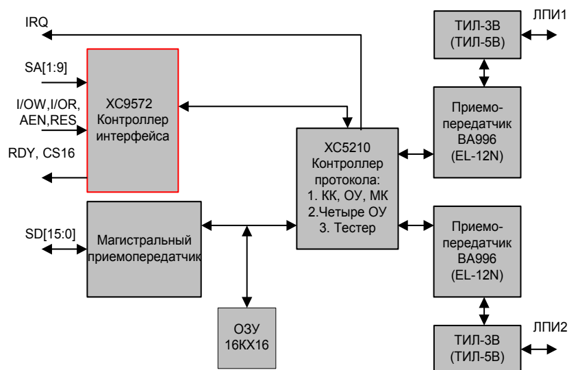
Рис. 1. Структурная схема
