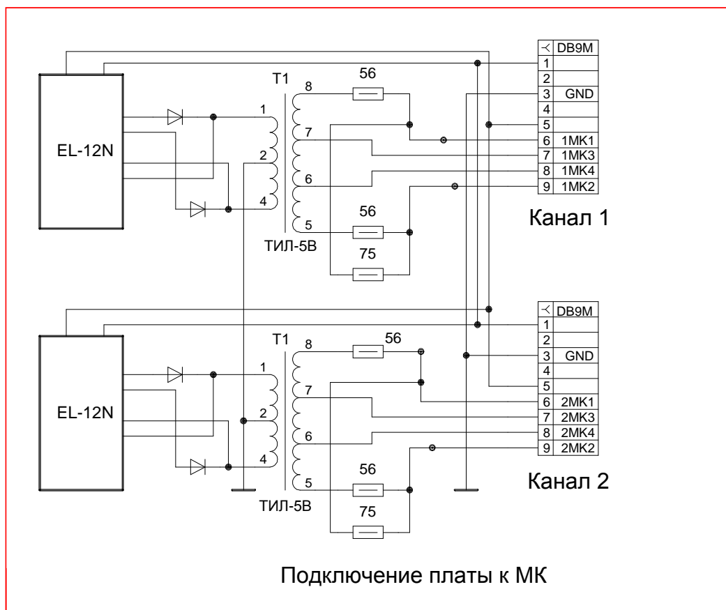
Рис.6 Подключение платы TX1-PC2 к линии передачи информации
