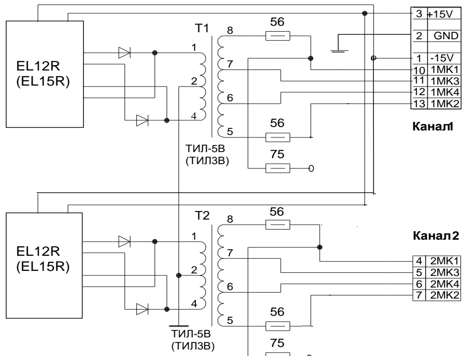
Подключение платы к МК ( вариант А )
