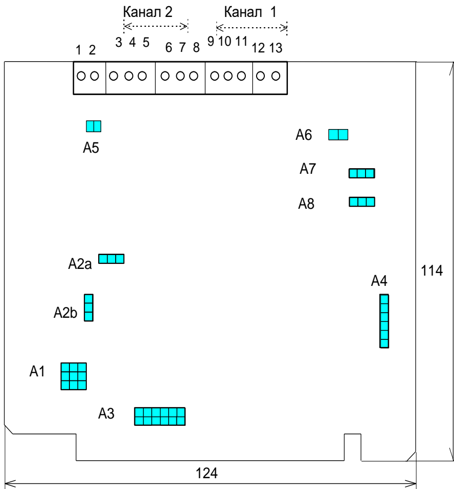
Рис.5а Условное изображение устройства ( вариант А)
