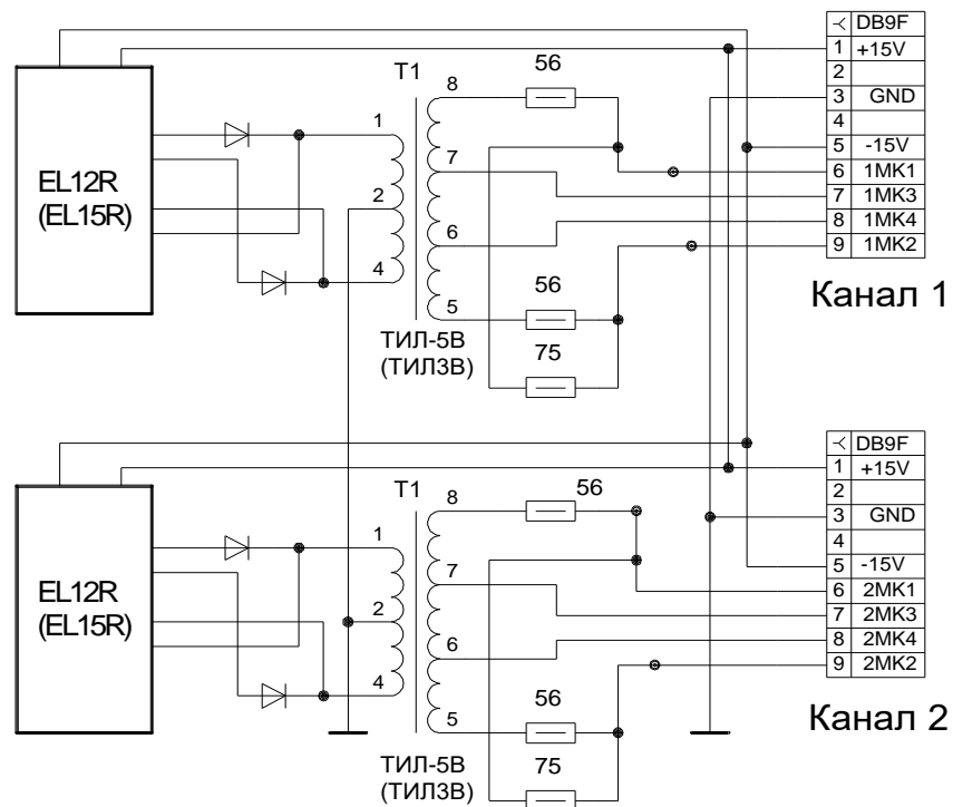
Подключение платы к МК ( вариант Б )
