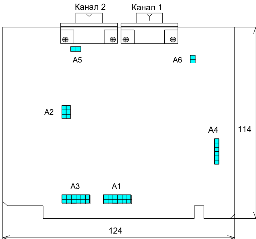
Рис.5б Условное изображение устройства ( вариант В)
