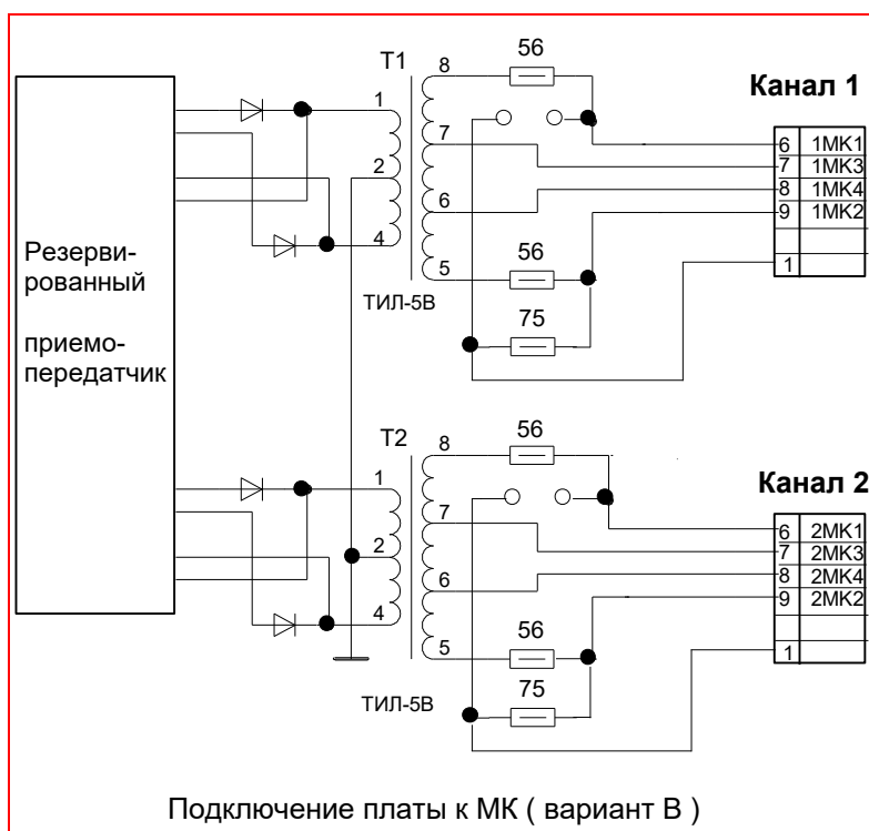
Рис.6 Подключение платы ТЕ1-МР к линии передачи информации
