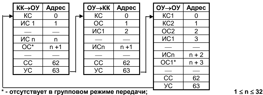
Рис. 4. Пример структуры блока памяти в режиме МТ.
