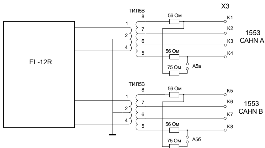
Рис. 6. Подключение устройства к линии передачи информации
