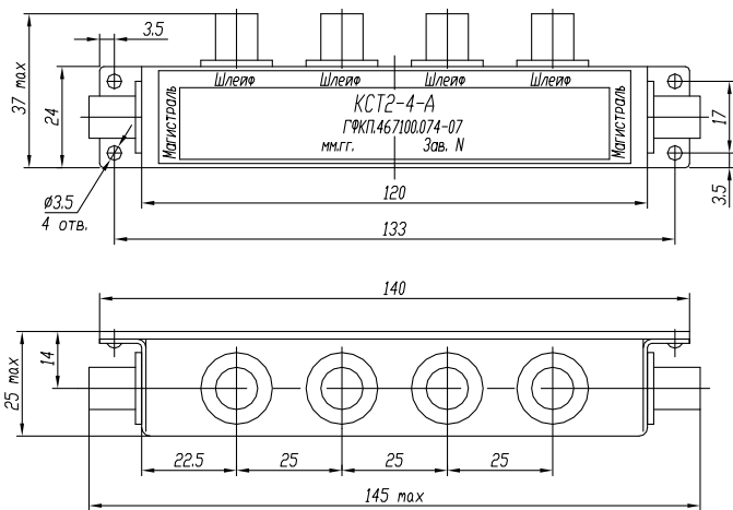
Габаритный чертеж коробки KCT2-4
