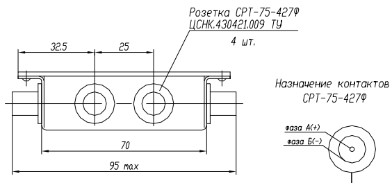
Габаритный чертеж коробки КСТ2-2
