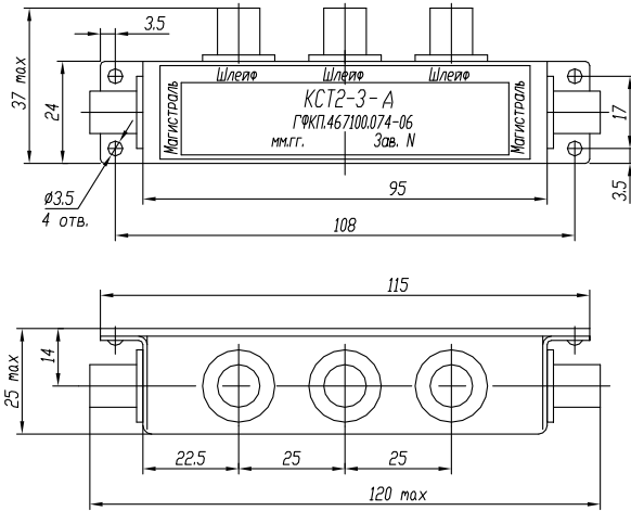
Габаритный чертеж коробки КСТ2-3
