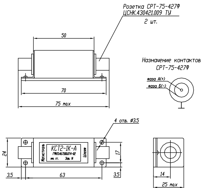
Габаритный чертеж коробки КСТ2-1К
