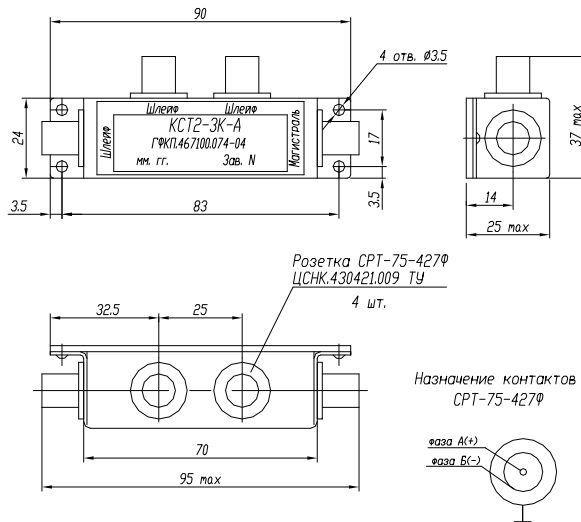
Габаритный чертеж коробки КСТ2-3К
