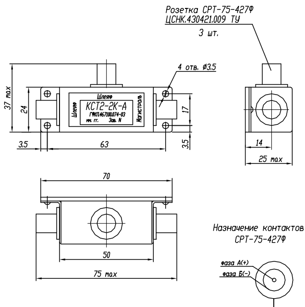
Габаритный чертеж коробки КСТ2-2К
