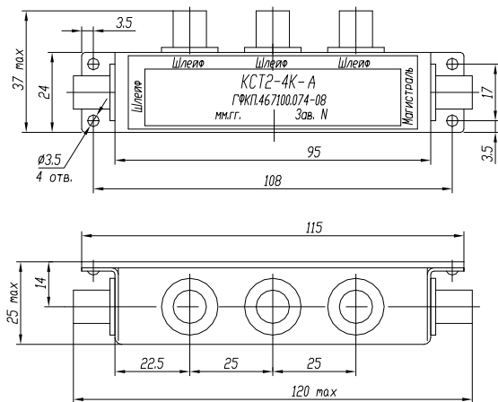
Габаритный чертеж коробки KCT2-4K
