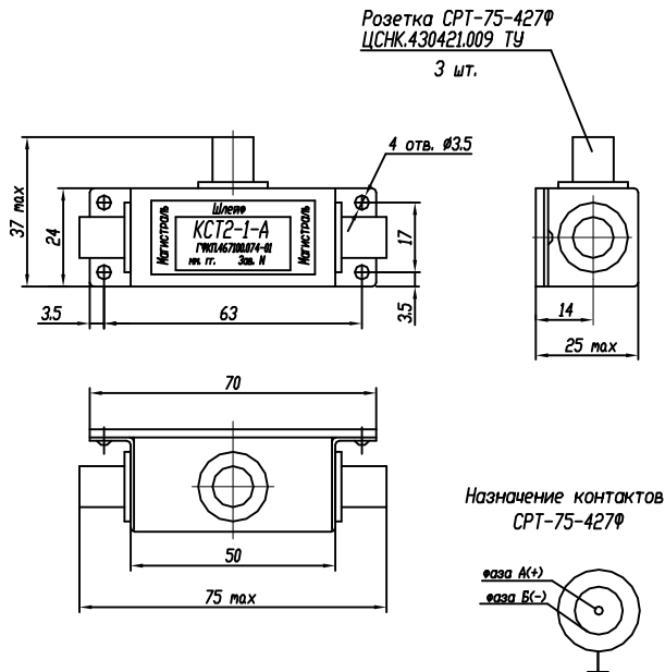
Габаритный чертеж коробки КСТ2-1
