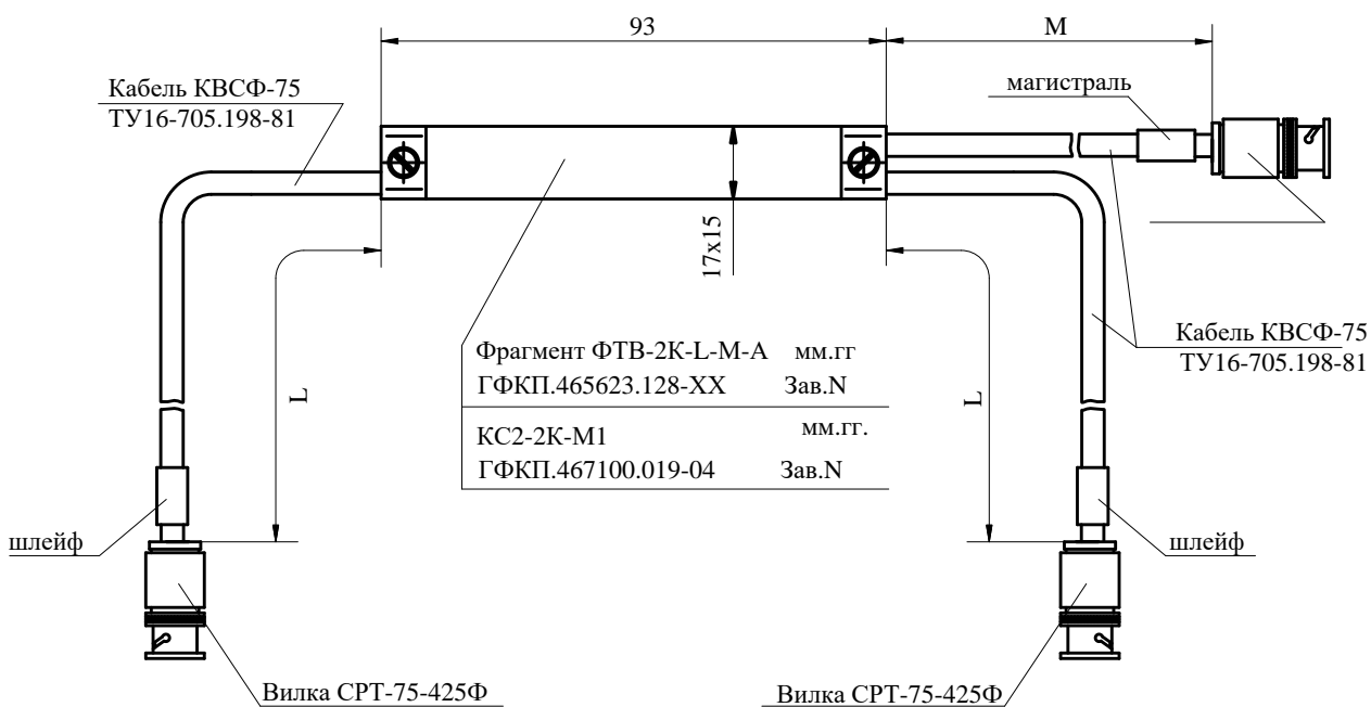
Габаритный чертеж фрагментов кабелей ФТВ-2К-L-M-A
