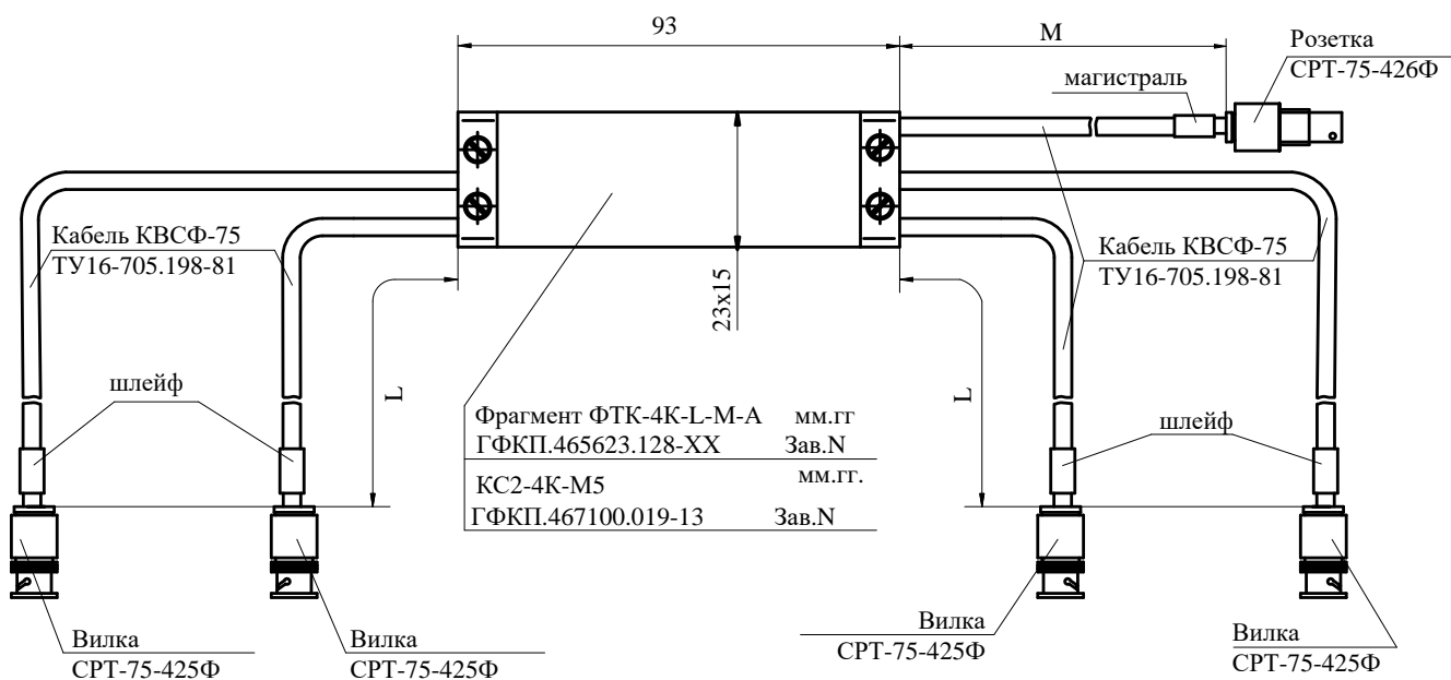
Габаритный чертеж фрагментов кабелей ФТК-4K-L-M-A
