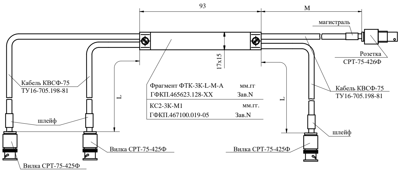
Габаритный чертеж фрагментов кабелей ФТК-3К-L-M-A
