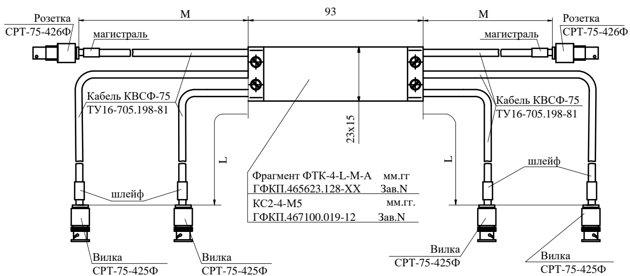
Габаритный чертеж фрагментов кабелей ФТК-4-L-M-A
