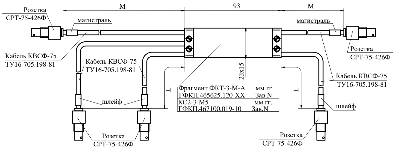
Габаритный чертеж фрагмента кабеля ФКТ-3-Л-М-А
