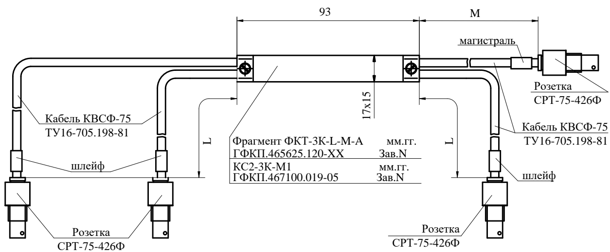
Габаритный чертеж фрагмента кабеля ФКТ-3К-Л-М-А
