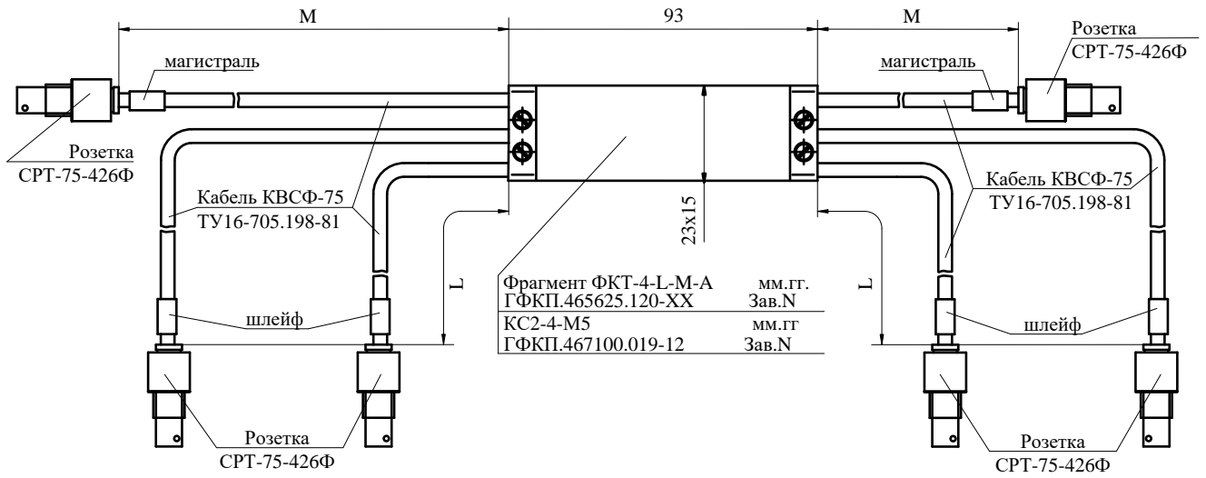
Габаритный чертеж фрагмента кабеля ФКТ-4-L-M-A
