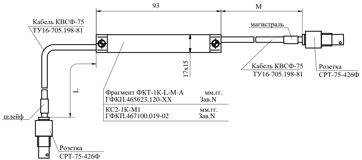
Габаритный чертеж фрагмента кабеля ФКТ-1К-L-M-A
