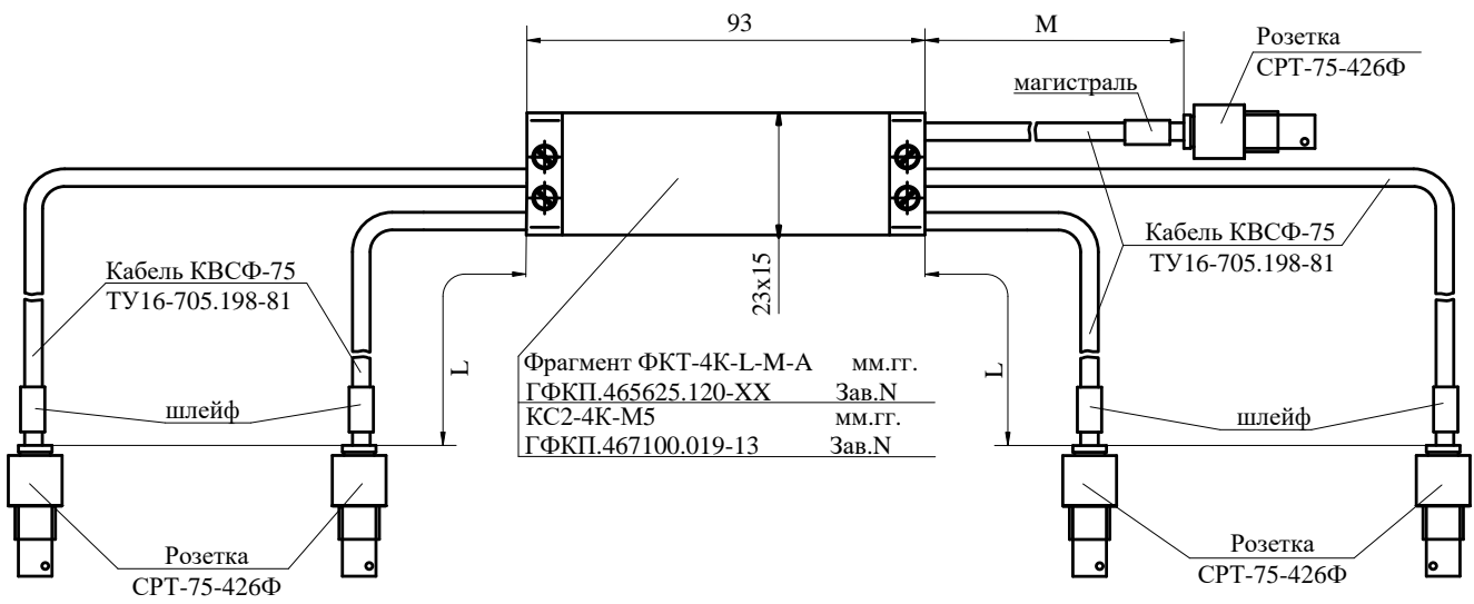
Габаритный чертеж фрагмента кабеля ФКТ-4K-L-M-A
