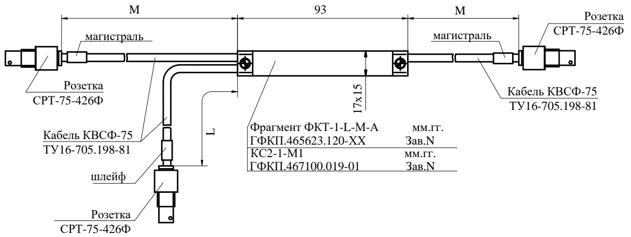
Габаритный чертеж фрагмента кабеля ФКТ-1-L-M-A
