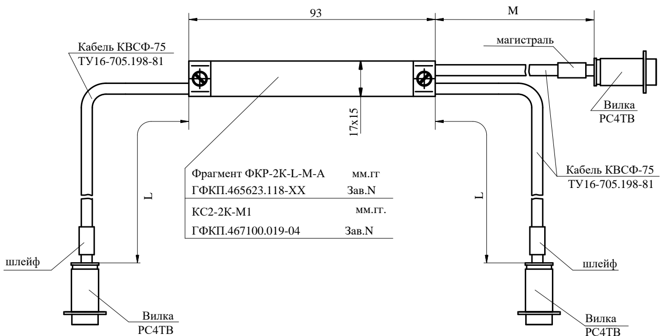
Габаритный чертеж фрагмента кабеля ФКР-2K-L-M-A
