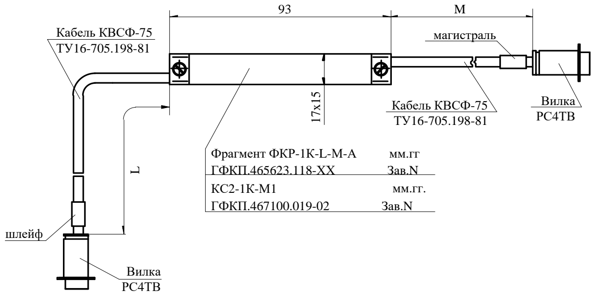
Габаритный чертеж фрагмента кабеля ФКР-1К-L-M-A
