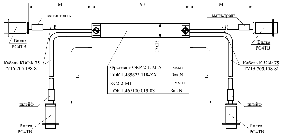
Габаритный чертеж фрагмента кабеля ФКР-2-L-M-A
