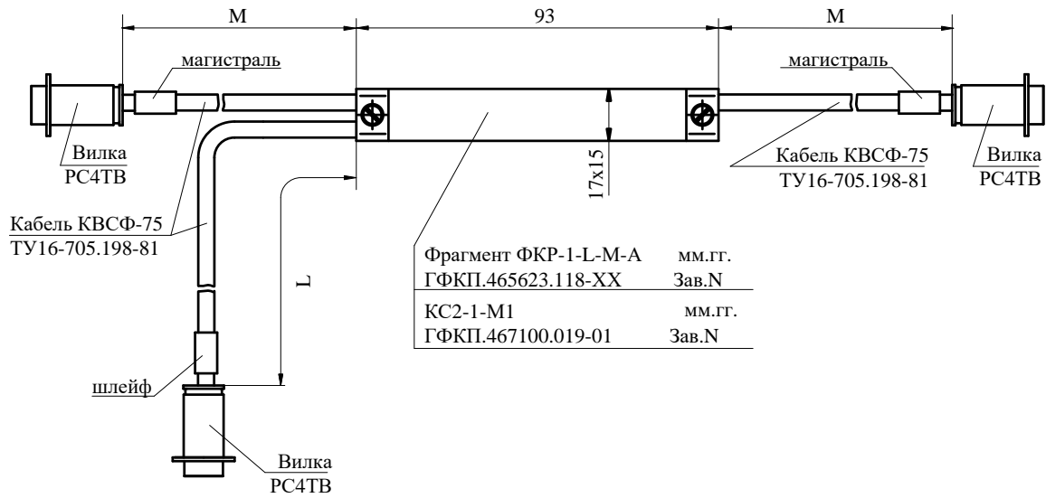
Габаритный чертеж фрагмента кабеля ФКР-1-L-M-A
