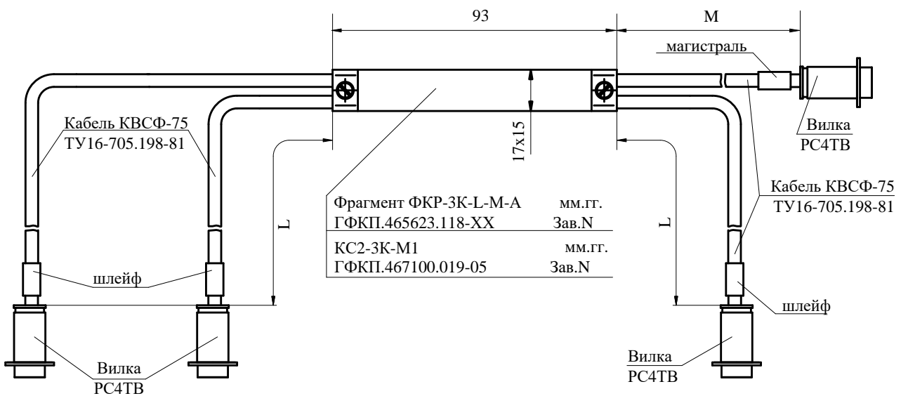
Габаритный чертеж фрагмента кабеля ФКР-3К-L-M-A
